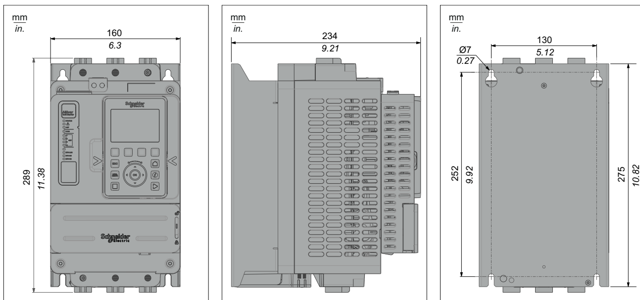
Vistas frontal, lateral y trasera
